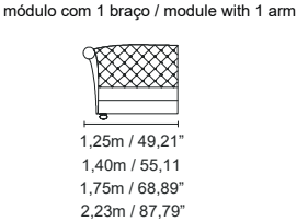
*Caixa com captonê. | *Box with tufting.
