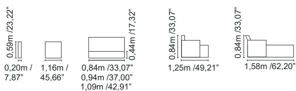
módulo fechado closed module
